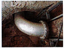
Mise en place du piquage et de la vanne d'isolement
