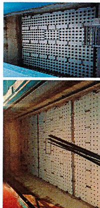
Mise en place du plancher
