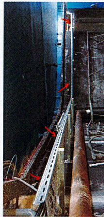
Chemins de câbles
